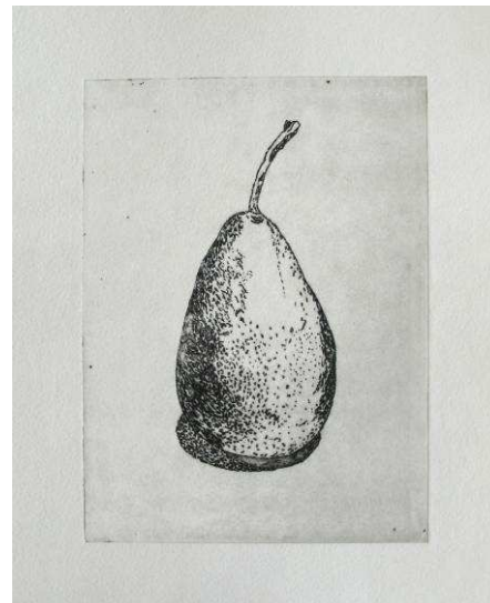
Une épreuve
