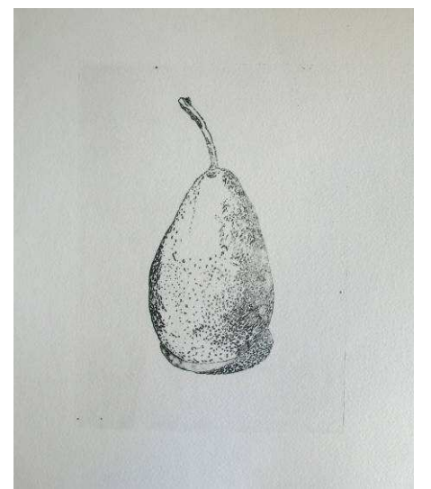
Une contre-épreuve
